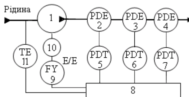
Рис. 1. Принципова схема гідродинамічного вимірювального перетворювача реологічних параметрів: 1 – задавач витрати; 2,3,4 – мостові гідродинамічні перетворювачі; 5,6,7 – дифманометричні перетворювачі; 8 – пристрій керування та обчислення; 9 – частотний перетворювач; 10 – асинхронний електродвигун; 11 – термоперетворювач.
