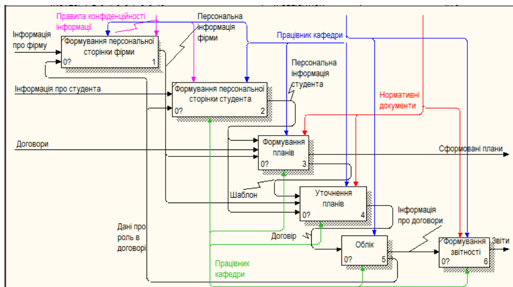
Рис. 1 - IDEF0 діаграма першого рівня декомпозиції.
