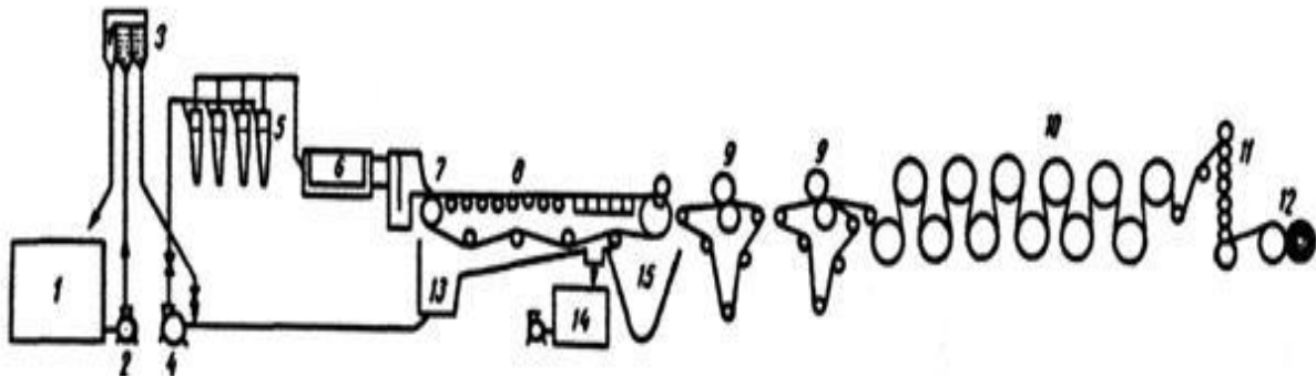
Рис. 1. Технологічна схема папероробної машини: 1 – акумулювальна ємність; 2 – масний насос; 3 – бачок переливу; 4 – змішувальний насос; 5 – вихрові очисники; 6 – вузлуловлювач; 7 – напірний ящик; 8 – сітковий стіл; 9 – мокрі преси; 10 – сушильна частина; 11 – каландр; 12 – накат; 13 – збірник оборотних вод; 14 – збірник надлишкових вод; 15 – басейн мокрого браку
