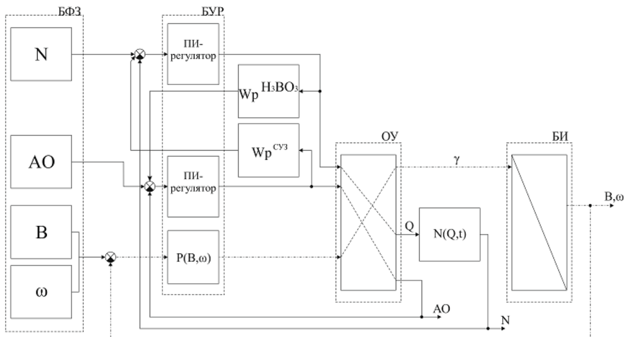
Рис. 1 Технологические основы автоматизированного управления
