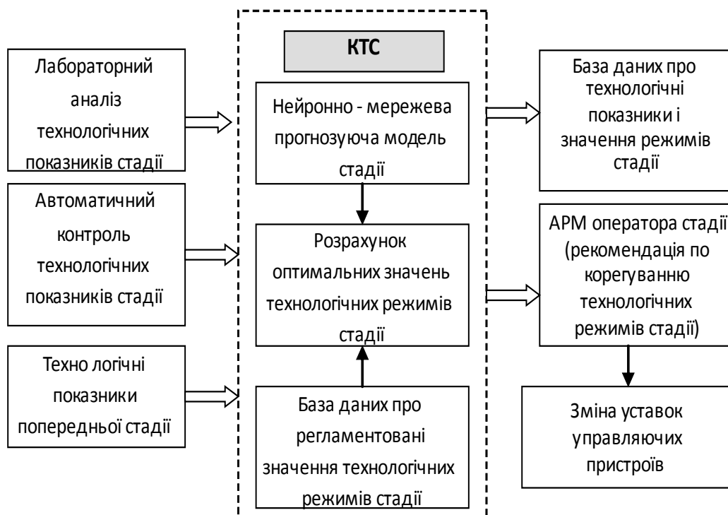
Рис.1. Структурна схема системи ПЕР для коригування технологічних режимів стадії виробництва хліба
