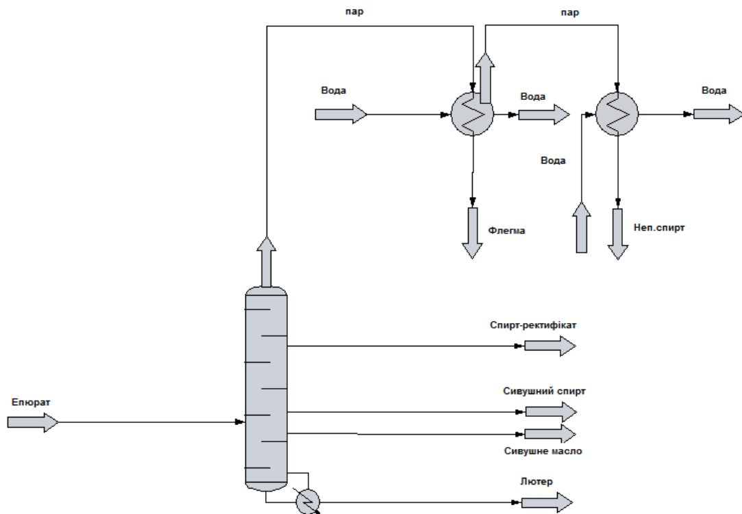
Рис. 1. Модель визначення флегмового числа колони та її впливу на концентрацію і кількісний склад продукту
