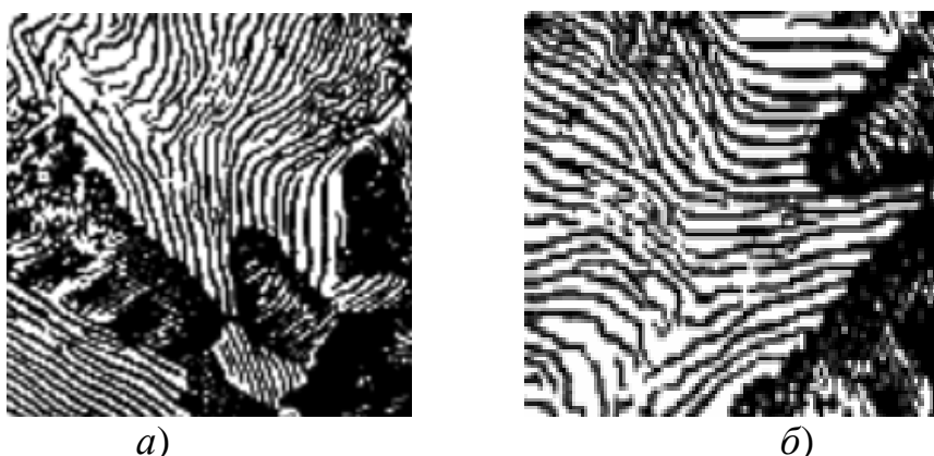
Рис. 1. Микроструктуры эвтектоидной стали (0,8 % углерода), содержащей пластинчатый перлит: a – D = 1,47 ; б – D = 1,21
