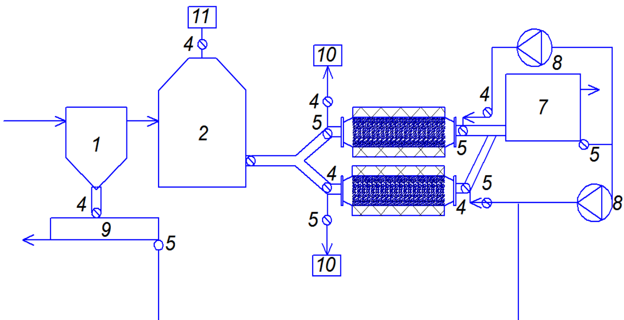
Рис. 1. Технологічна схема очистки нафтовмісних стічних вод
