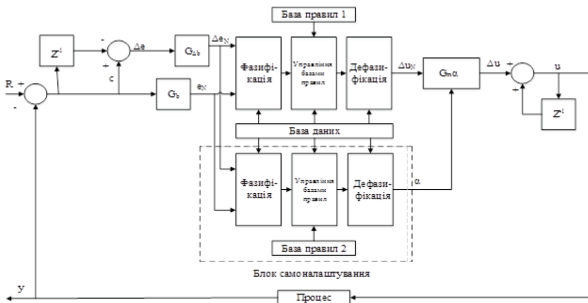
Рис. 1. Нечіткий ПІ контролер з самоналаштуванням (СННПК)
