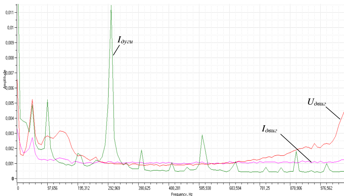
Рис. 1. Осциллограммы спектральной плотности I_{\text{дуги}}(t) , I_{\text{якоря}}(t) , U_{\text{якоря}}(t) на частотах от 0 до 1 кГц
