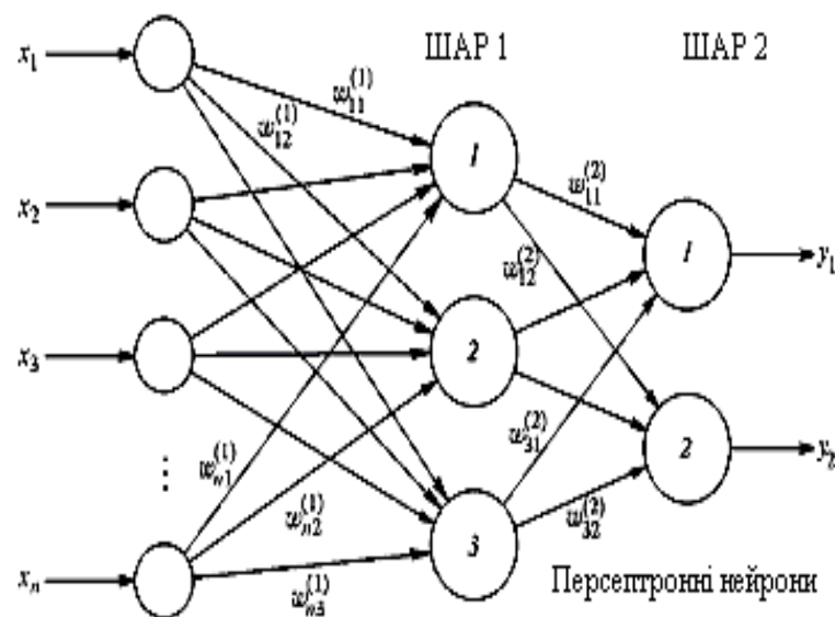
Рис. 1. Двошаровий персептрон
