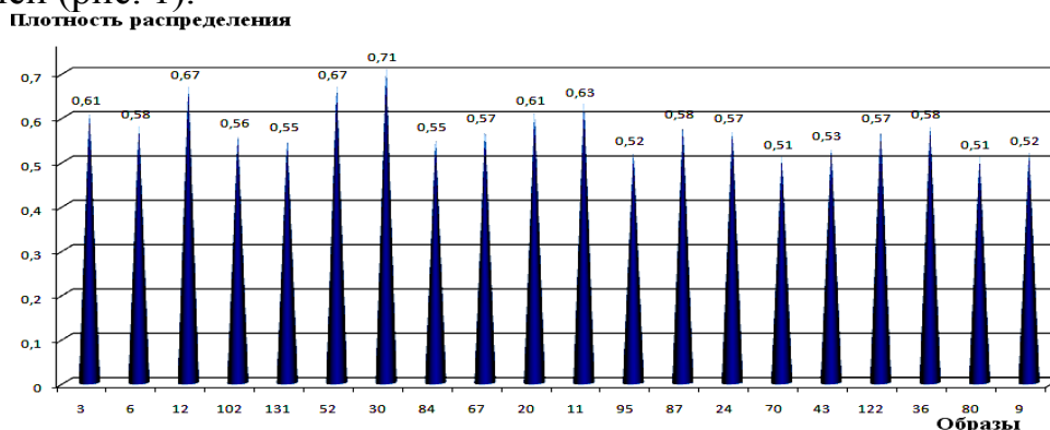
Рис. 1. Плотности распределения при определении температурных образцов
